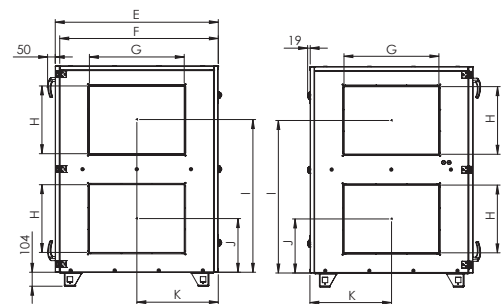
Duoblock (VEX1030RS - VEX1080RS)
