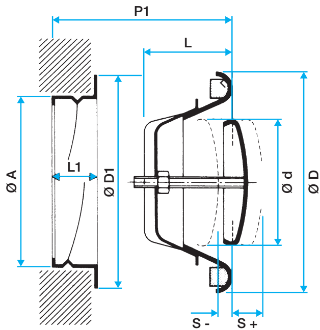
Bouche SR 143 avec manchette
