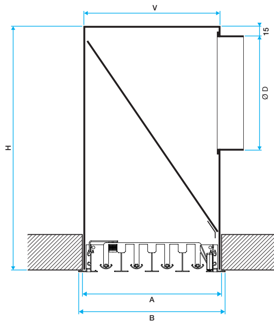
Lined E Slim avec plénum. Fixation S2
