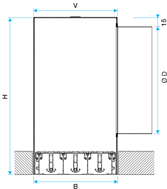
Lined Combined Standard Ouvrant Côté Reprise
