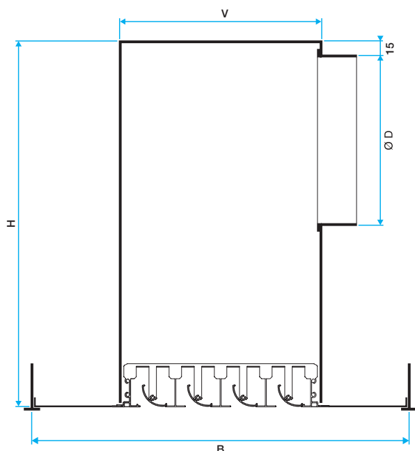
Lined Combined Standard Ouvrant Côté Reprise
