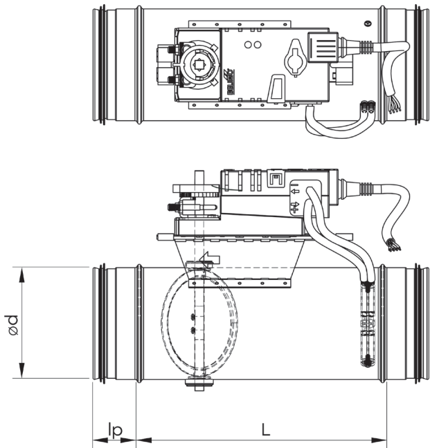
Maßskizze (Standard-Ausführung)
