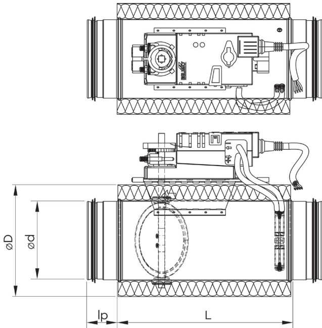
Maßskizze (Isolierte Ausführung)
