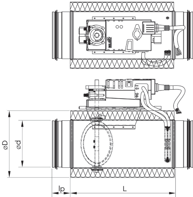
Maßskizze (Isolierte Ausführung)
