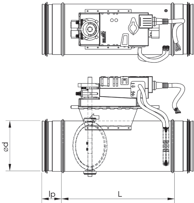
Maßskizze (Standard-Ausführung)
