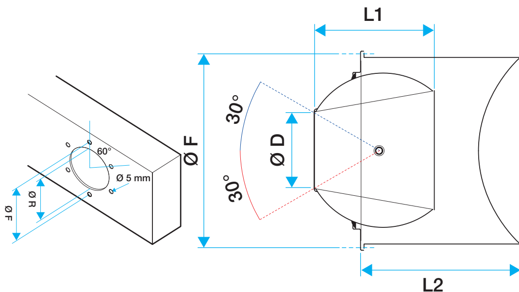
Diffuseur AR 190 - Montage sur gaine rectangulaire
