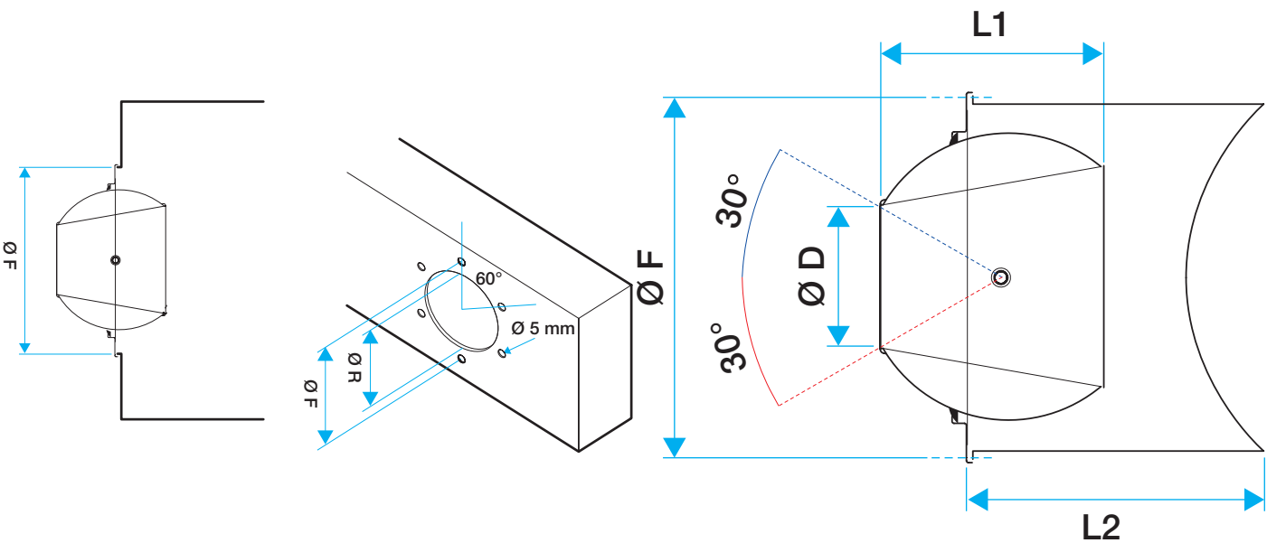
Diffuseur AR 190 - Montage sur gaine rectangulaire
