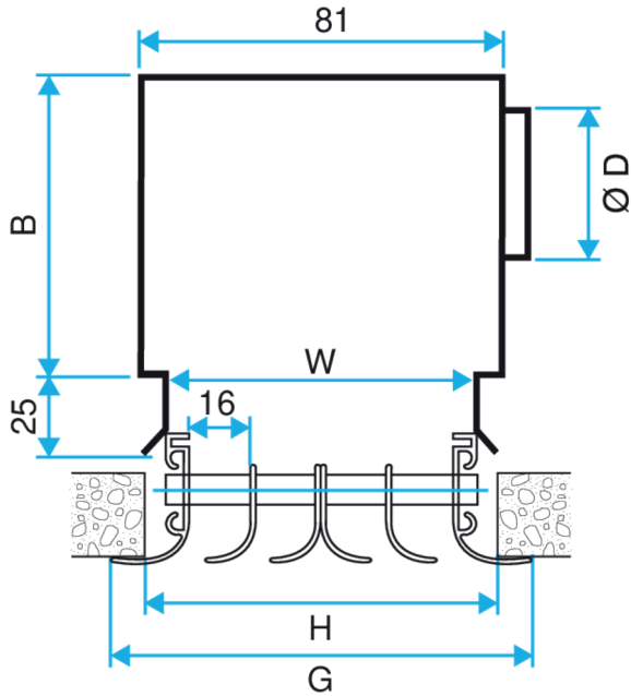
Diffuseur ALD 610 - 620
