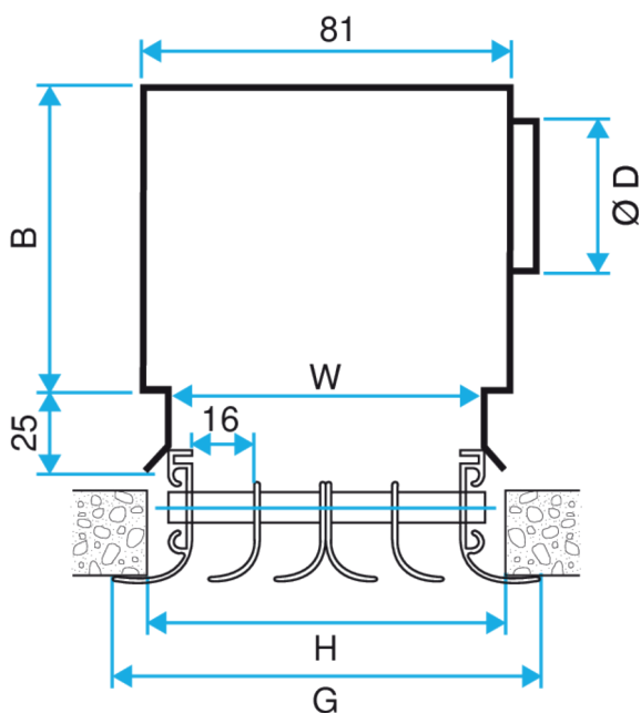
Diffuseur ALD 610 - 620
