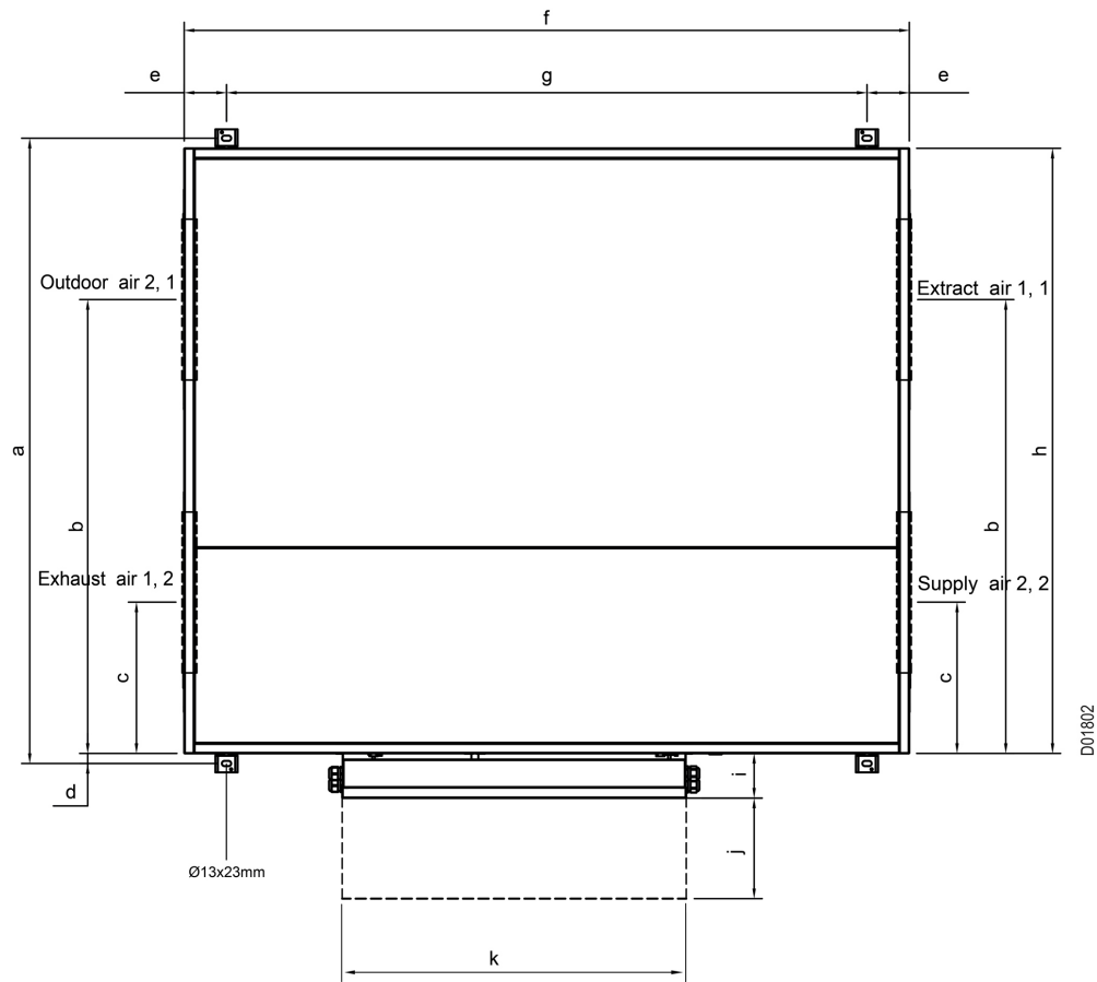
Ansicht von oben CX3030L/CX3040L/ CX3050L/CX3060L
